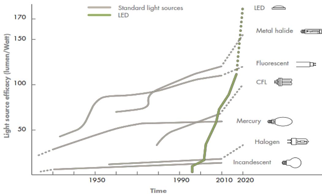
شکل ۳. مقایسه بهره نوری LED و سایر منابع نوری استاندارد در طی زمان
