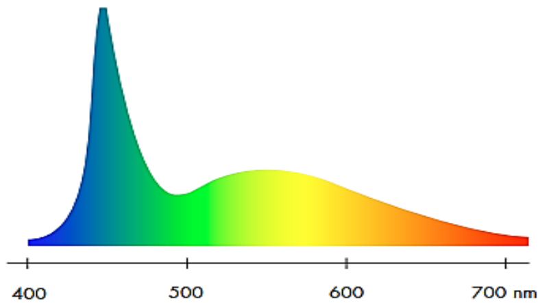
شکل ۲. توزیع توان طیفی LED (میزان نور منتشر شده در هر طول موج) به روش تبدیل فسفری.
